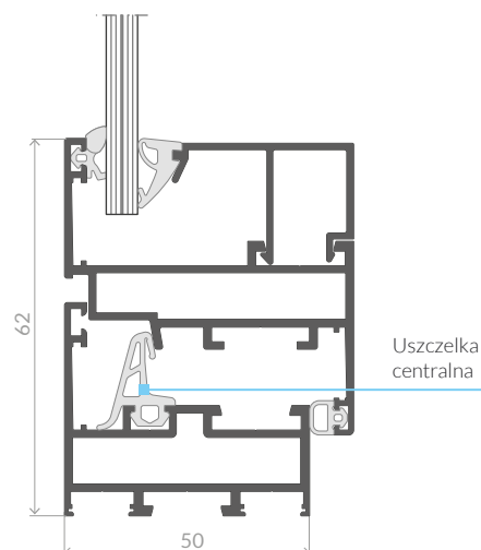
Przekrój przez okno otwierane
